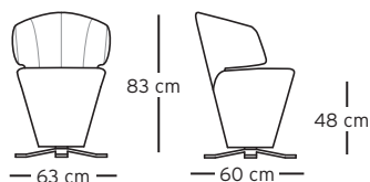
Stuhl mit Sternfuß Chair with star base
