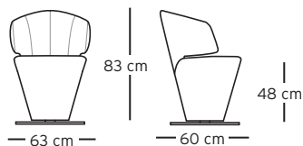
Stuhl mit Drehteller Chair with revolving base
