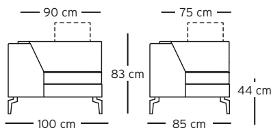
3 links 3 left Abschlusselemente links End elements left
